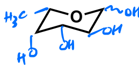
Fuc
