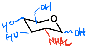
GlcNAc
