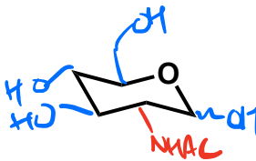
GalNAc
