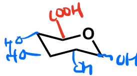
GlcUA
